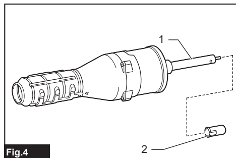
Fig. 4 ► 1. Pipe 2. Cap
