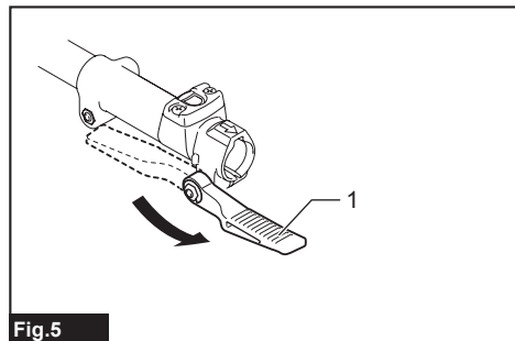
Fig. 5 ► 1. Lever
